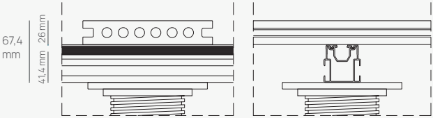
Sistema con rastreles de aluminio con banda amortiguadora sobre plots · System with aluminium battens with shock absorbing strips on plots · Système de lattes en aluminium avec bandes d'absorption des chocs sur les parcelles · Система с алюминиевой обрешеткой с амортизирующими планками на участках
