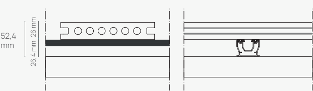
Sistema con rastreles de aluminio con banda amortiguadora. System with aluminium batten with shock-absorbing strip. Système avec bande d'aluminium avec bande d'absorption des chocs. Система с алюминиевыми рейками с амортизирующей лентой.
