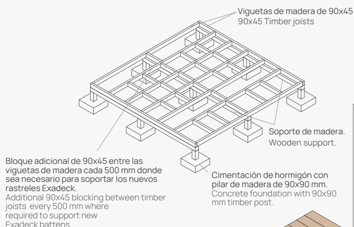
ESTRUCTURA DE MADERA EXISTENTE EXISTING DECK SUBFLOOR STRUCTURE
