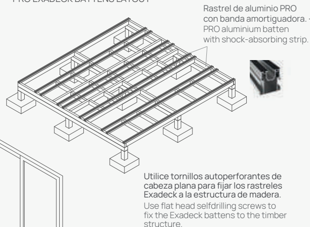
ESTRUCTURA DE RASTRELES PRO EXADECK PRO EXADECK BATTENS LAYOUT
